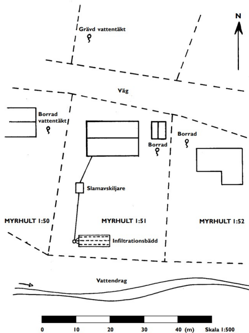
Exempel på situationsplan med enskild avloppsanläggning
